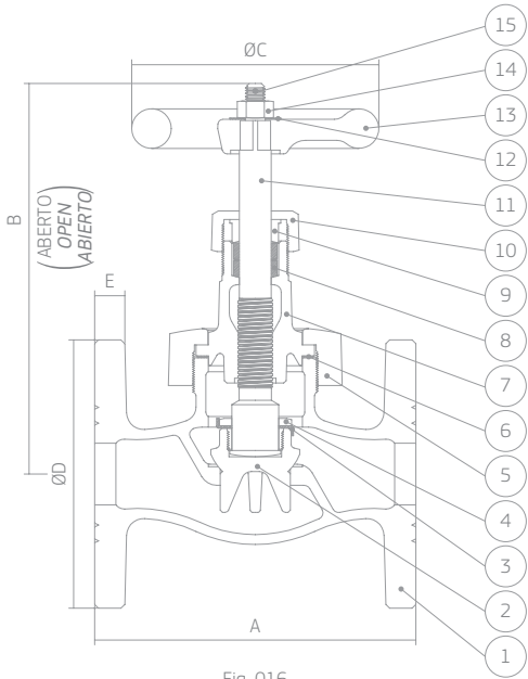
Fig. 016 Disco metálico mettalic disc disco metálico
