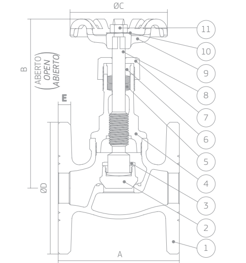
Fig. 013 Disco metálico metallic disc disco metalico
