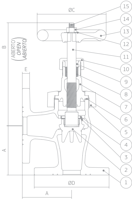
Fig. 030 Disco metálico mettalic disc disco metálico
